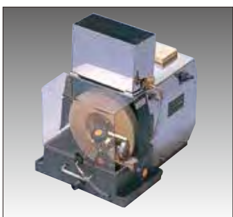
⑬ 自動研磨機スーパークラウン E-8 直 納3 /100V・200W 寸法:350×250×355 1台 ¥197,000 661-7200 ※中砥石付
