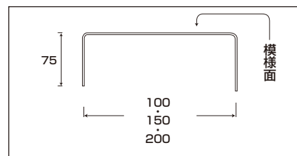
⑦ アイスダミー E-4 納5
