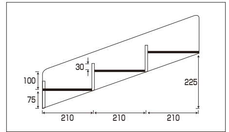
③ ボトルヒナ段 E-9 納4 寸法・600×630×175 1台 ¥23,600 213-4010 材質・アクリル5mm
