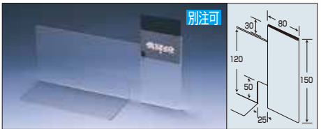
④ 見出しホルダー仕切板 E-3 納4
