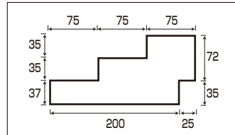
⑥ スライドヒナ段 N-7 直 寸法・350~685×225×107 /元払・15台 1台 ¥2,900 213-1106 材質・PS/色・クリア、白、黒
