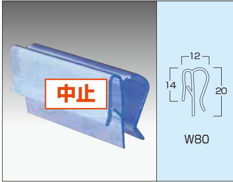
① イージークリップF型 E-16 在 1袋(100入) 411-1006 材質・エンビ
