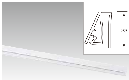
⑧ プライスカードホルダー白 E-16 納3 寸法・1000×23 1本 ¥1,200 222-0123 ご希望の寸法でカット致します(最大1000mmまで)寸法と 個数、ご連絡ください。御見積りいたします / 材質・エンビ
