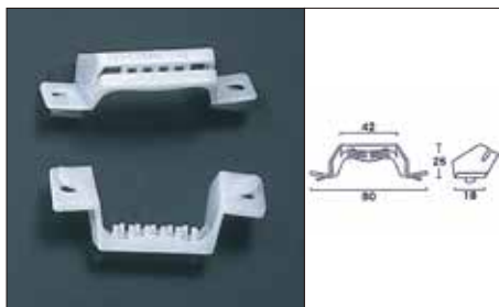
⑦ 冷ケースポップ立 E-16 在 寸法・80×18 1個 ¥220 411-5845 材質・POM
