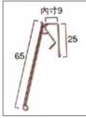
① スウィングライナー-V3 フックタイプ E-14 直
