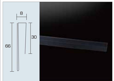
⑤ PETロングカード差し(0.5mm) C-15 納4
