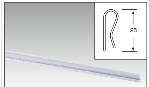
⑨ オリジナル引掛 大 透明 E-16 納3 寸法・1500×25 1本 ¥740 222-0124 ご希望の寸法でカット致します(最大1500mmまで) 寸法と個数、ご連絡ください 御見積りいたします / 材質・エンビ
